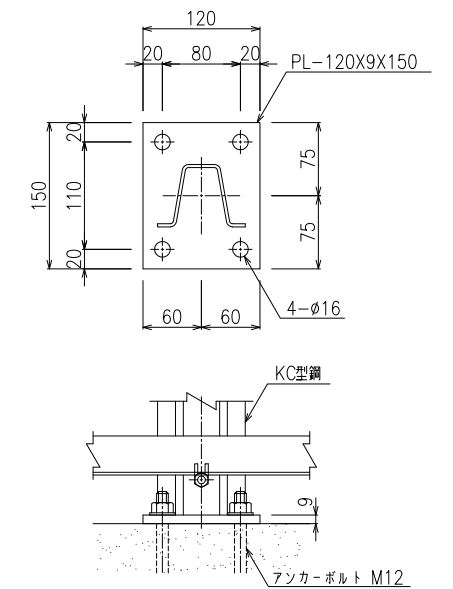
基礎部取付詳細図 S=1/4
