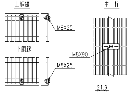
メッシュ取付部 S=1/6
