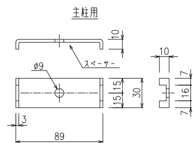
取付金具詳細図 S=1/2
