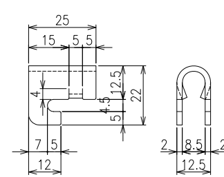
胴縁取付金具 S=1/1
