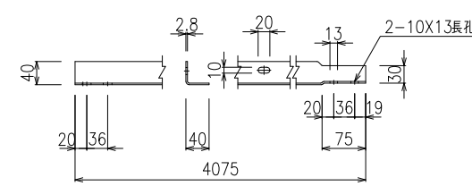
下胴縁
