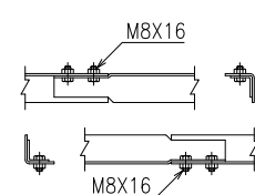
胴縁継手部 S=1/6
