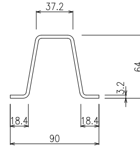
主柱 S=1/2
