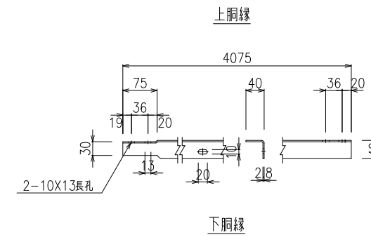
胴縁詳細図 S=1/6
