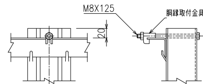
取付金具詳細図 S=1/2
