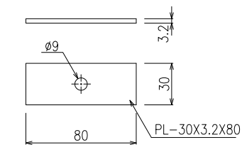
スペーサー
