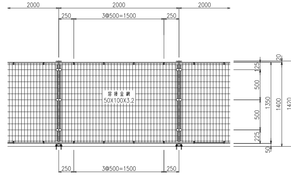
正面図 S=1/20
