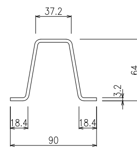
主柱 S=1/2
