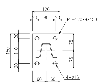
基礎部取付詳細図 S=1/4
