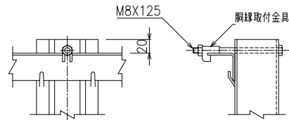
主柱胴縁取付部 S=1/4
