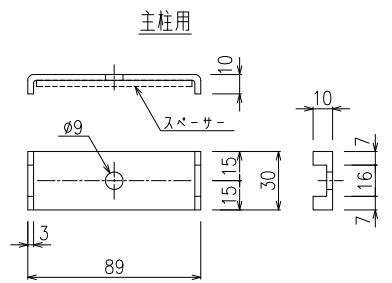
スペーサー
