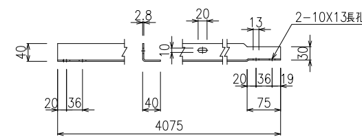
下胴縁
