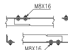
胴縁継手部 S=1/6
