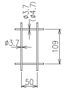
メッシュ寸法図 S=1/5
