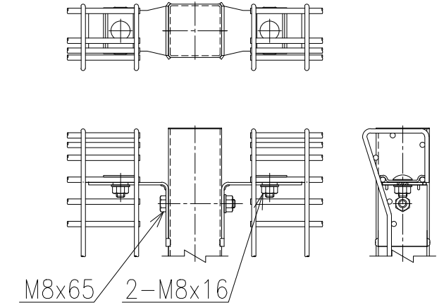
C部詳細図 S=1/5
