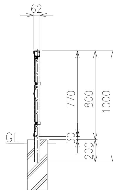
側面図 S=1/20
