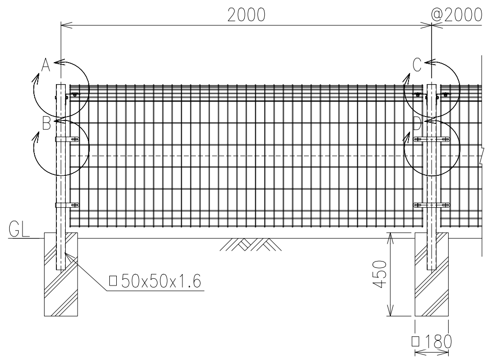
正面図 S=1/20
