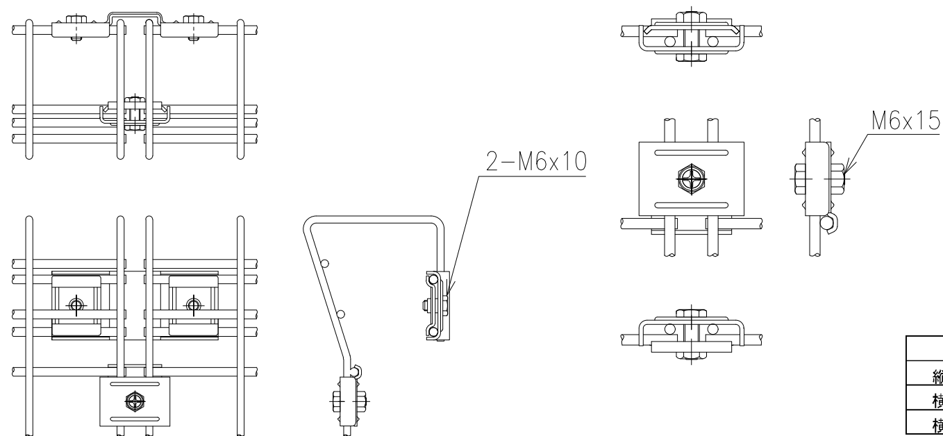
B部詳細図 S=1/3
