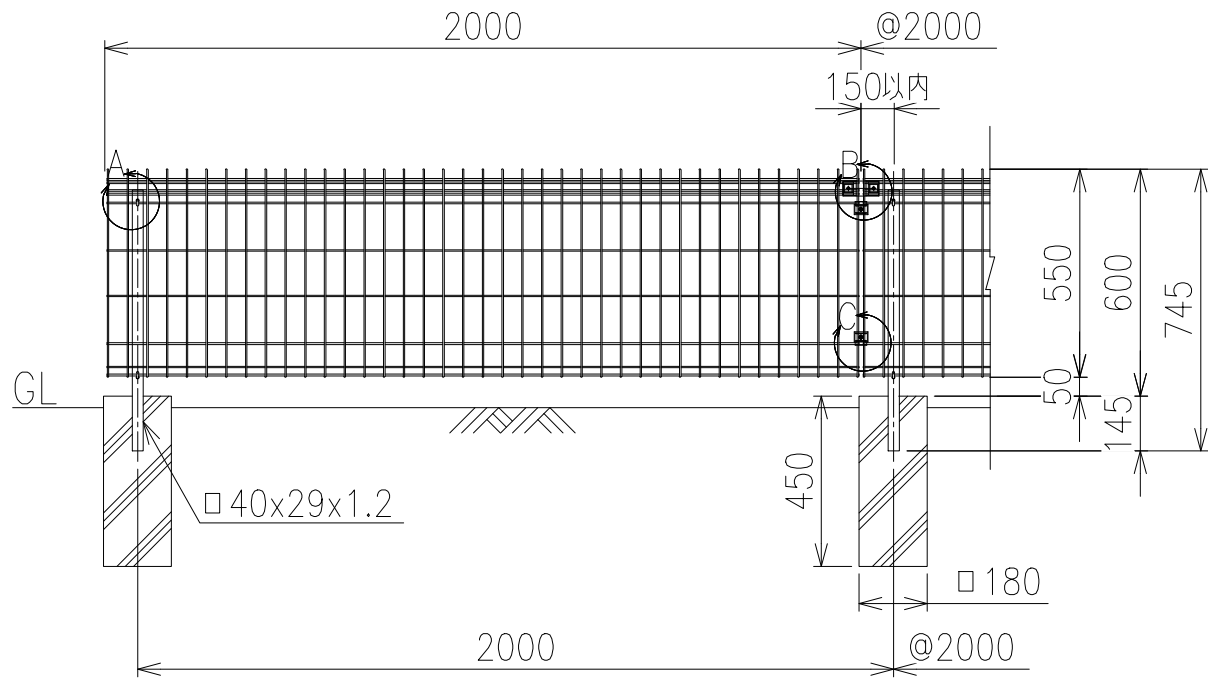
正面図 S=1/20
