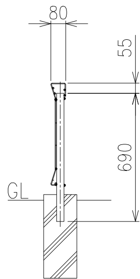
側面図 S=1/20
