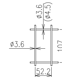
メッシュ寸法図 S=1/5
