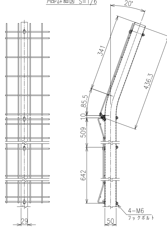
A部詳細図 S=1/6
