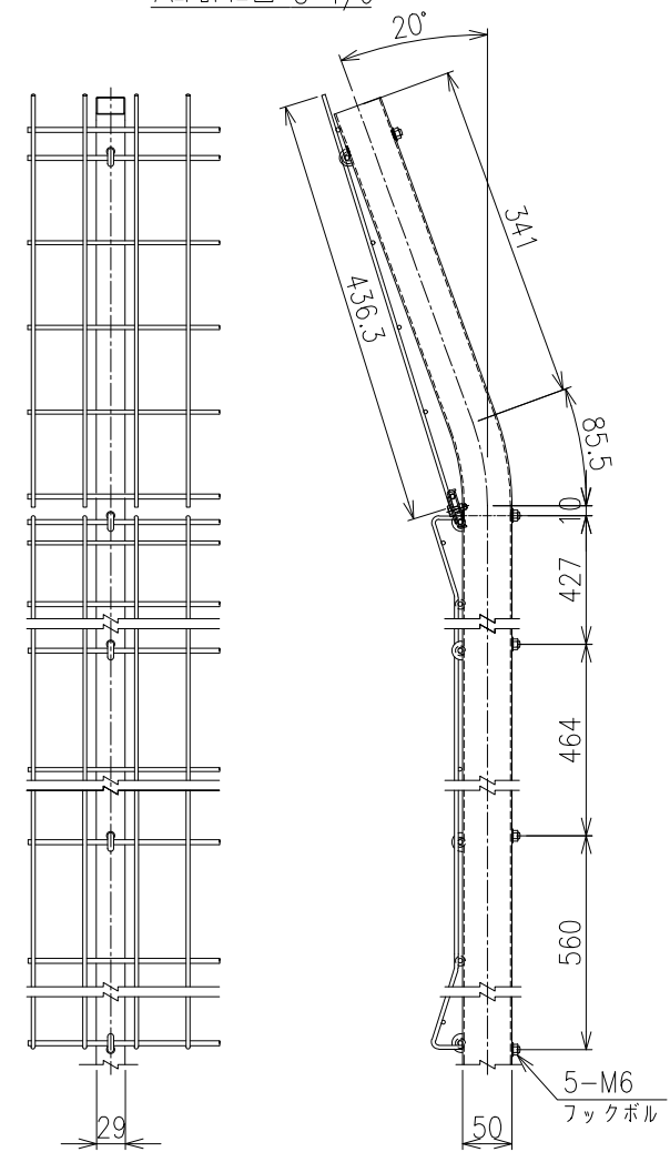
A部詳細図 S=1/6
