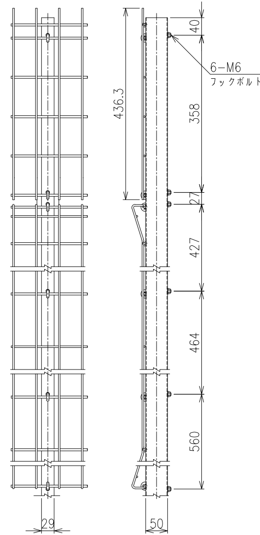
忍び部分 メッシュ寸法図 S=1/5
