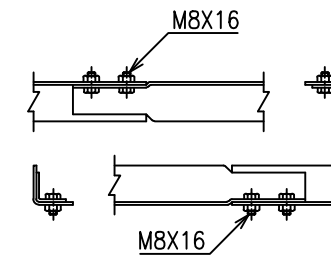
胴縁継手部 S=1/5
