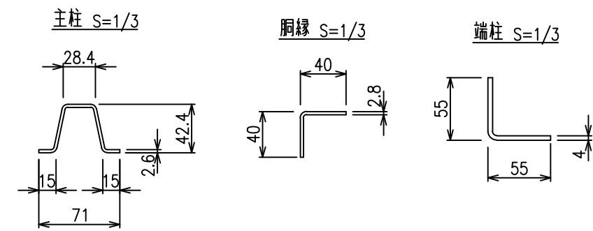
取付金具類詳細図
