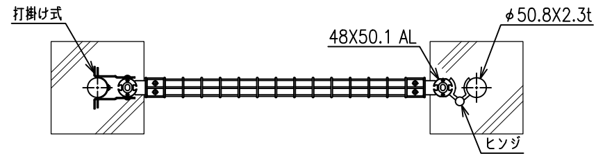
片開き門扉 (H-120・W-102)
