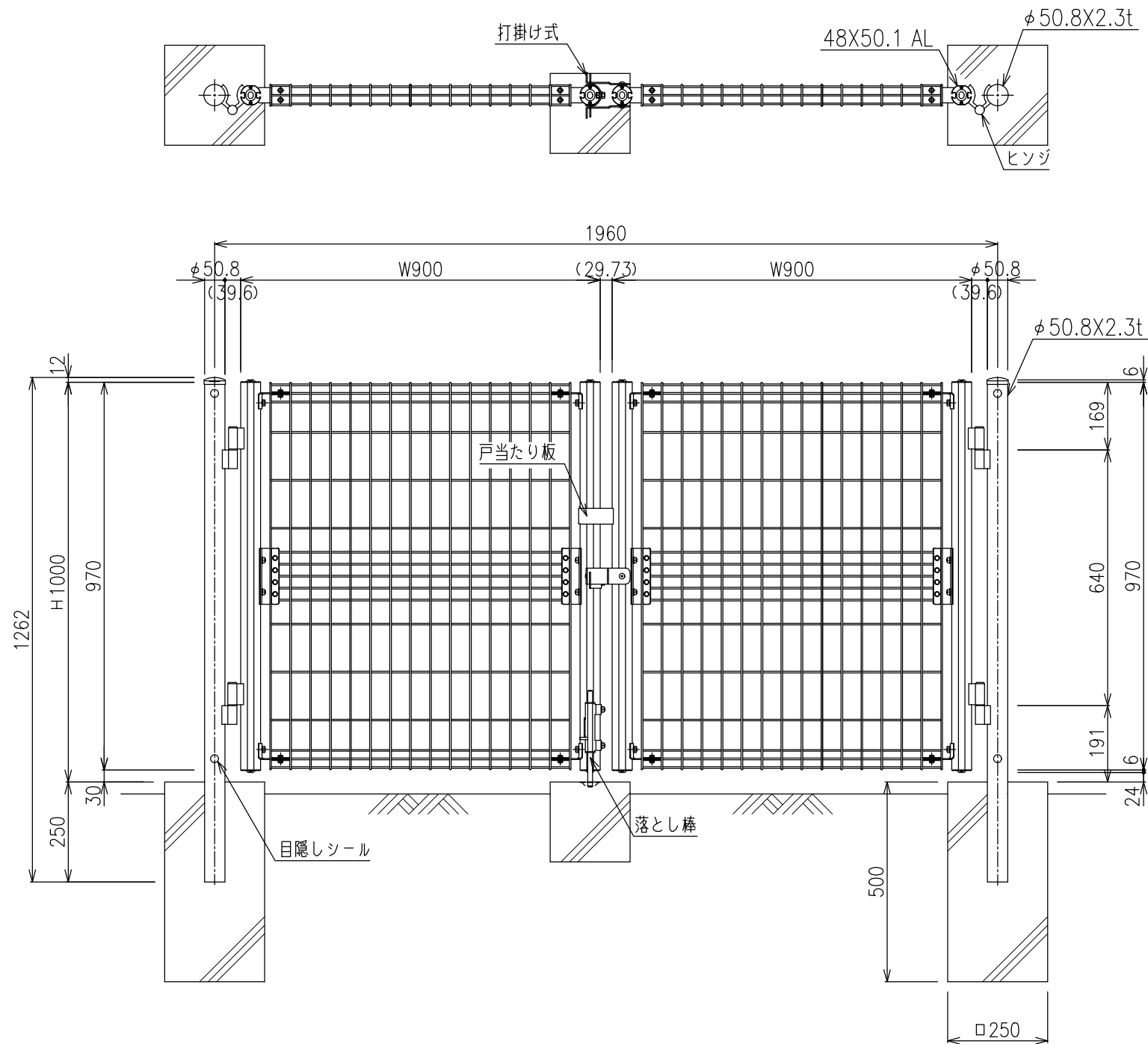
両開き門扉 (H-100・W-196)
