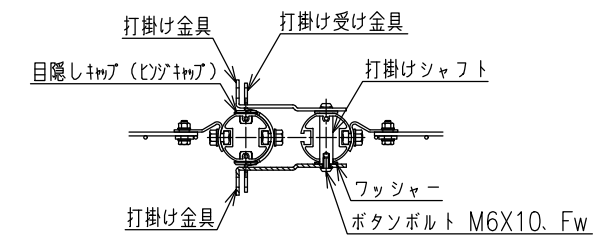
両開打掛部詳細図
