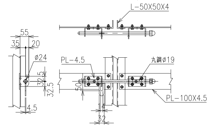
施錠詳細図 S=1/10
