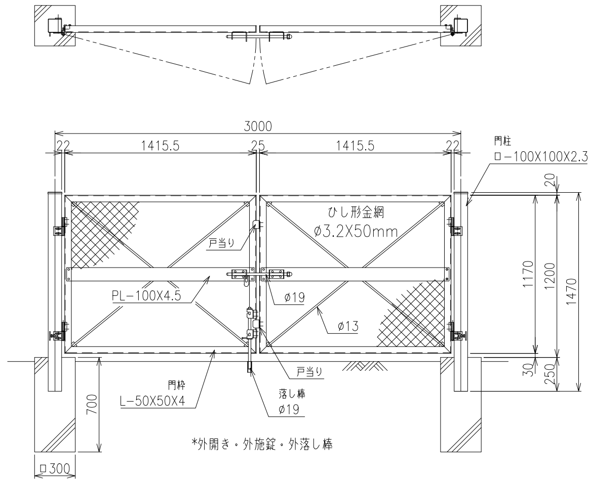
両開き門扉 S=1/20 H-120,W-300
