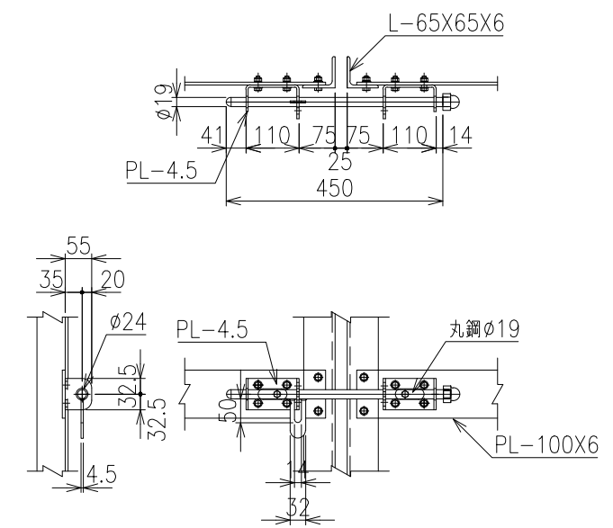
施錠詳細図 S=1/10
