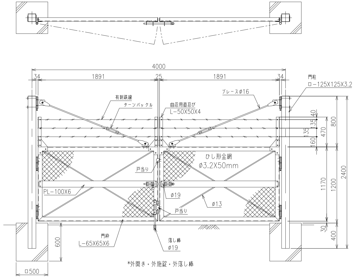
両開き門扉 S=1/20 H-120,W-400
