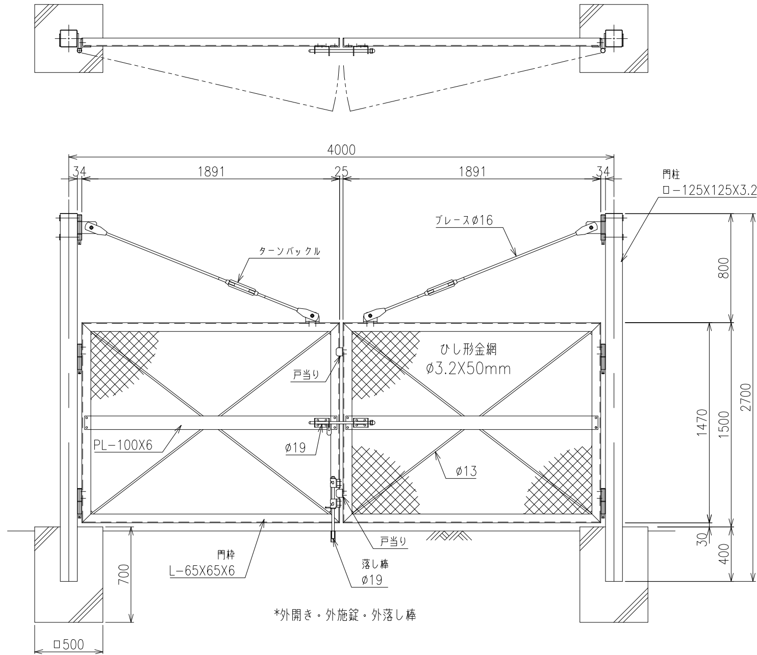
両開き門扉 S=1/20 H-150,W-400
