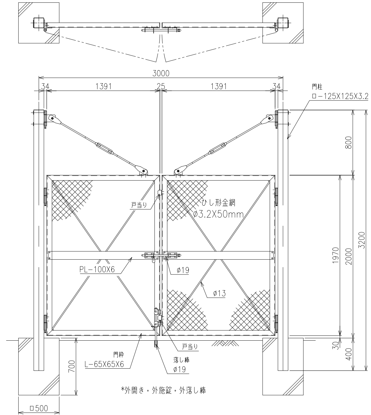
両開き門扉 S=1/20 H-200,W-300
