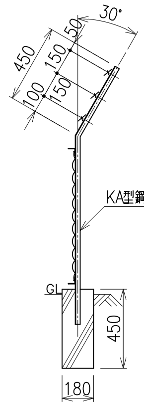
側面図 S=1/20
