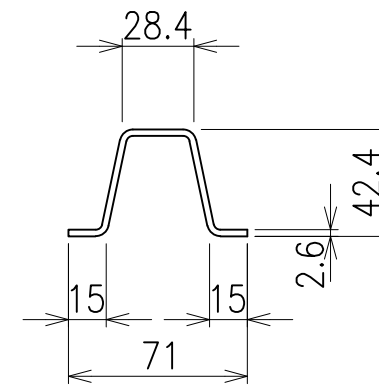
主柱 S=1/3
