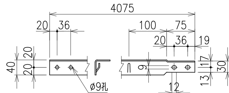
胴縁 S=1/6
