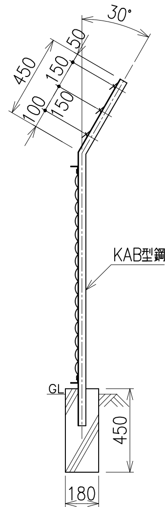
側面図 S=1/20
