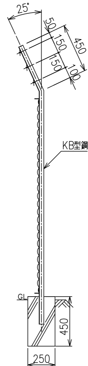
側面図 S=1/20
