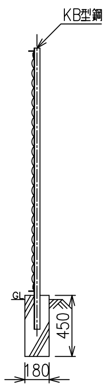
側面図 S=1/25
