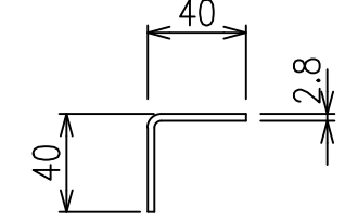
胴縁 S=1/3
