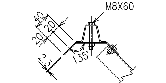
コーナー柱と胴縁取付部 S=1/5
