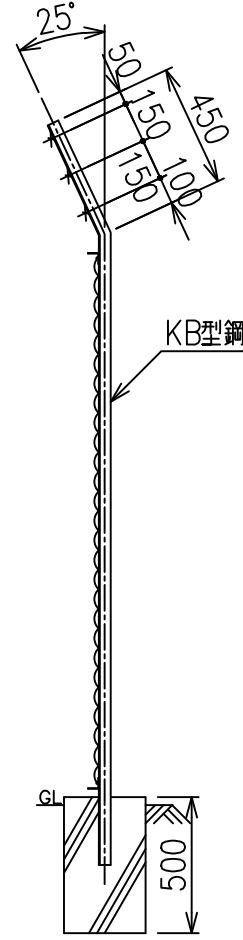
側面図 S=1/25
