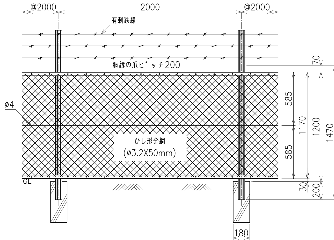
正面図 S=1/20
