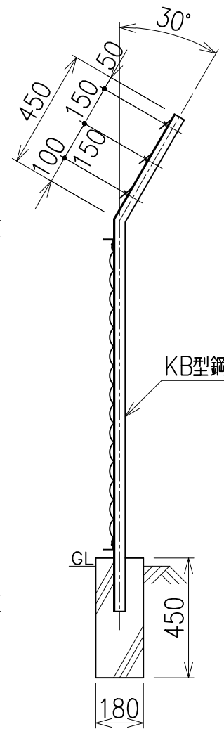
側面図 S=1/20
