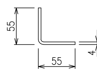
端柱断面図 S=1/3
