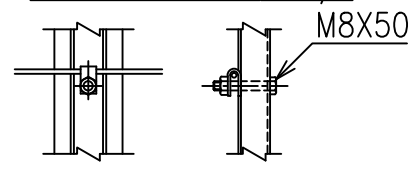
胴縁継手部 S=1/6
