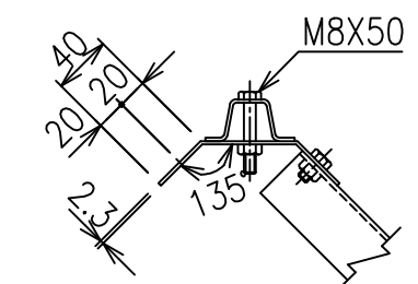
コーナー柱と胴縁取付部 S=1/5
