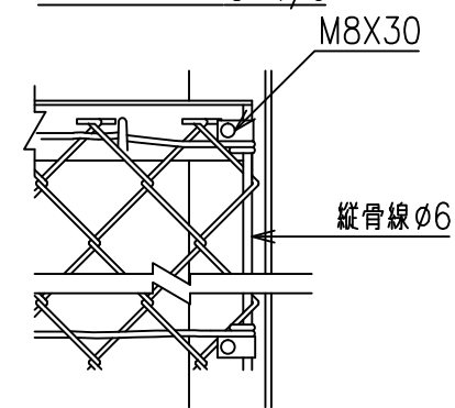
胴縁 S=1/6
