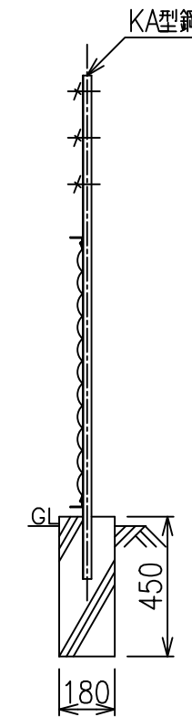
側面図 S=1/20
