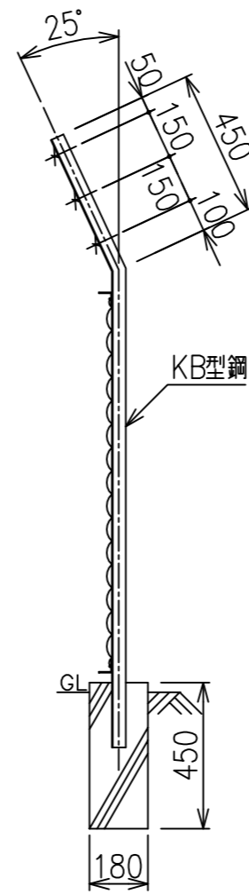
側面図 S=1/20
