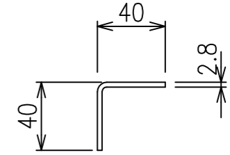
胴縁 S=1/3
