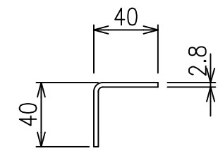
胴縁 S=1/3
