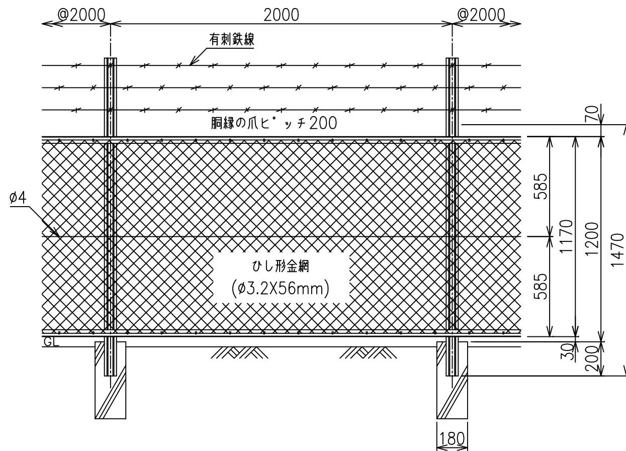
正面図 S=1/20
