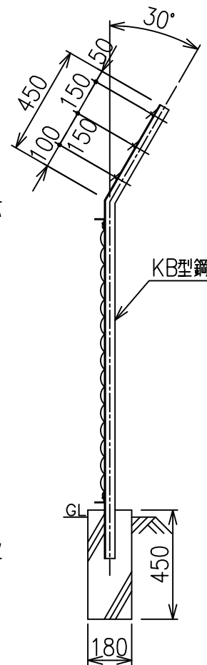
側面図 S=1/20
