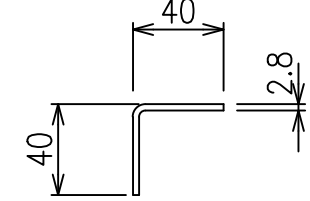
胴縁 S=1/3
