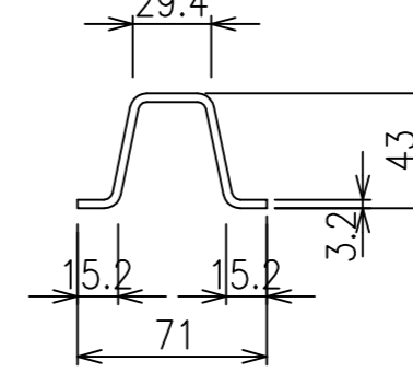
主柱 S=1/3
