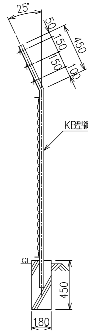
側面図 S=1/20
