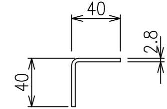
胴縁 S=1/3
