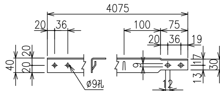
胴縁 S=1/6
