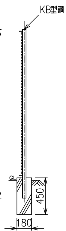
側面図 S=1/25
