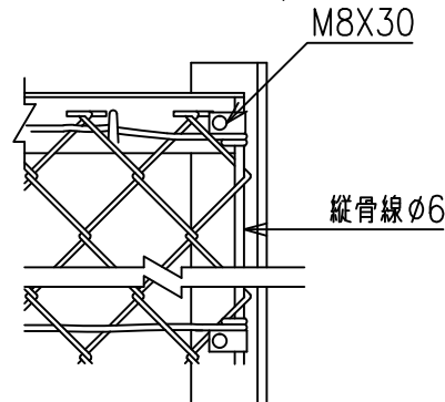
胴縁 S=1/6
