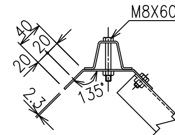
コーナー柱と胴縁取付部 S=1/5
