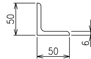
端柱断面図 S=1/3
