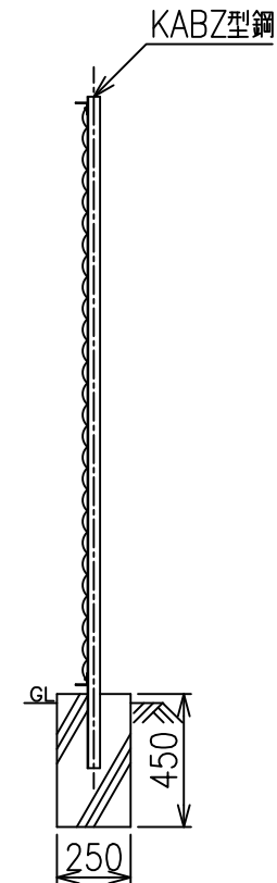
側面図 S=1/25
