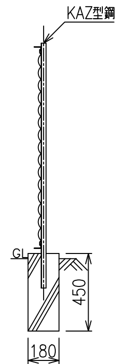
側面図 S=1/20
