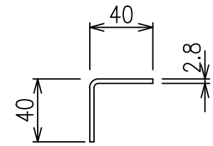
胴縁 S=1/3
