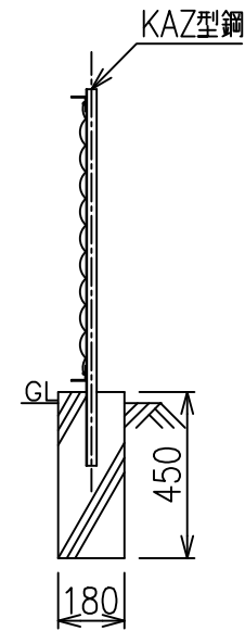
側面図 S=1/20
