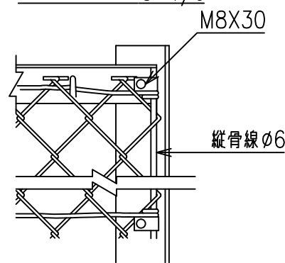
胴縁 S=1/6
