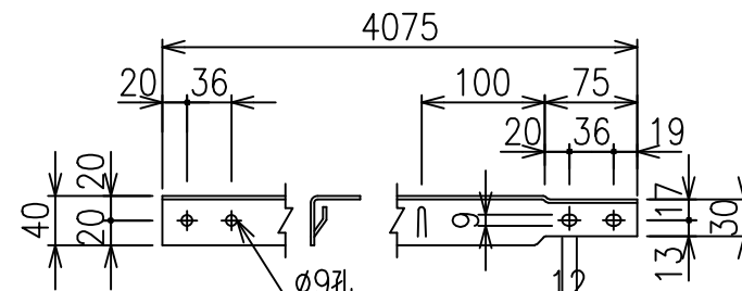
胴縁 S=1/6
