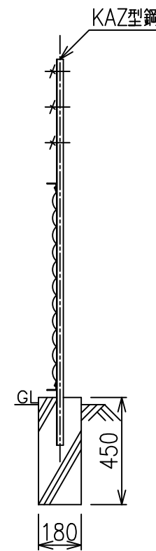
側面図 S=1/20
