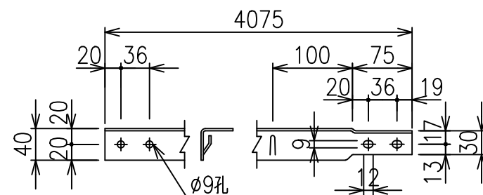
胴縁 S=1/6
