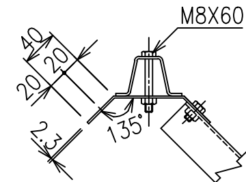
コーナー柱と胴縁取付部 S=1/5
