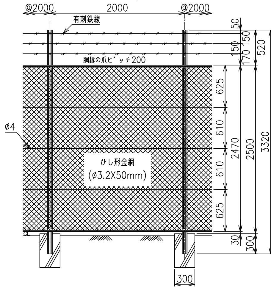
正面図 S=1/30
