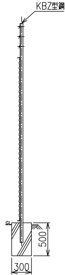
側面図 S=1/30
