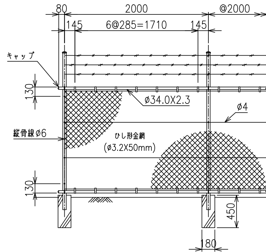
組立図 S=1/30
