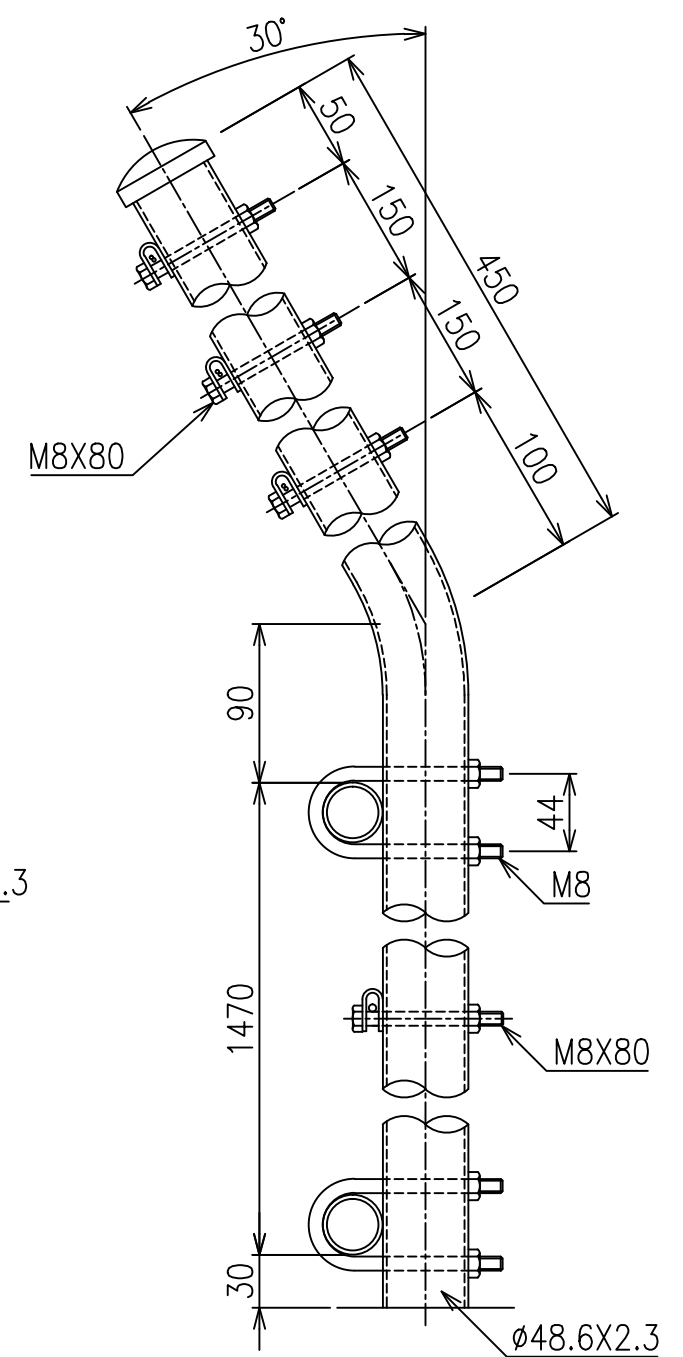
胴縁骨線取付詳細図 S=1/4
