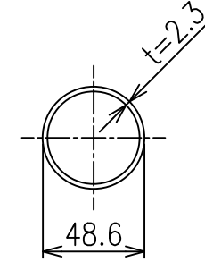
主柱 S=1/3
