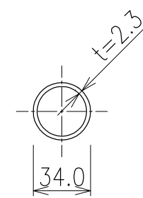
胴縁 S=1/3
