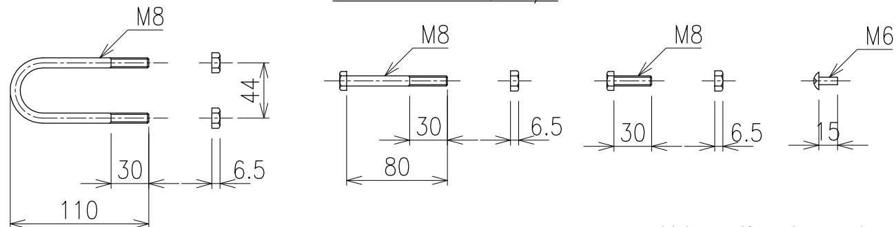
ボルトナット S=1/4
