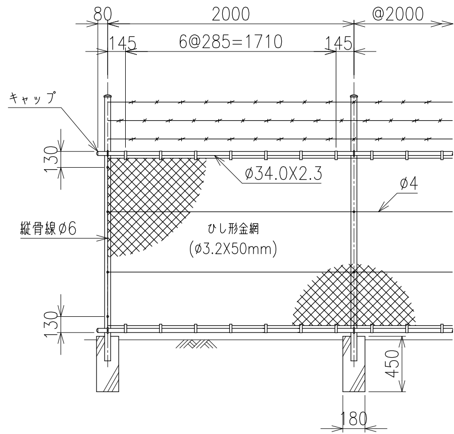
組立図 S=1/30
