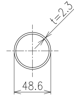
主柱 S=1/3
