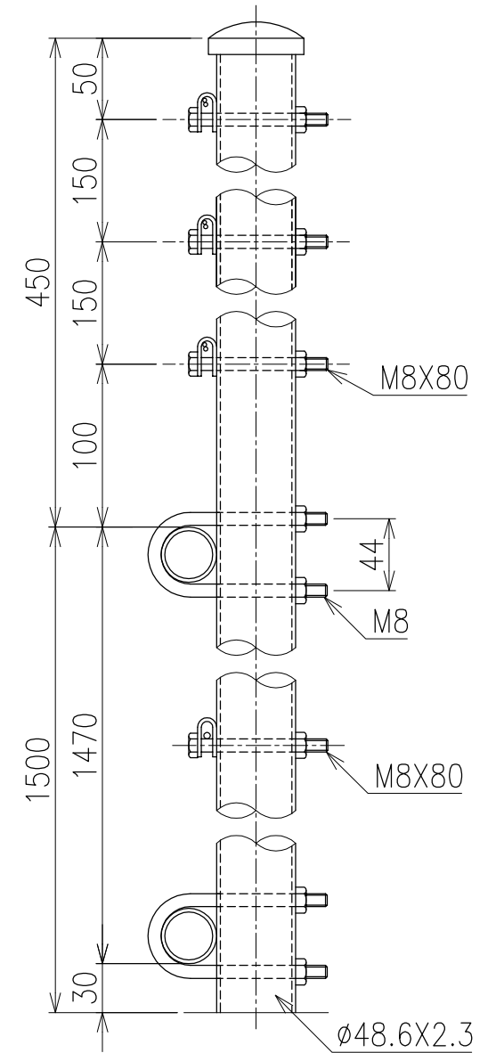
胴縁骨線取付詳細図 S=1/4
