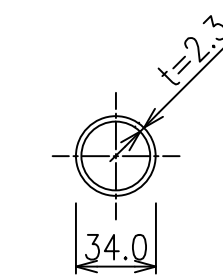
胴縁 S=1/3
