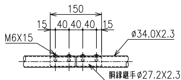
胴縁継手詳細図 S=1/6
