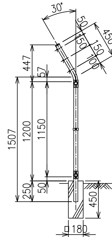
側面図 S=1/25
