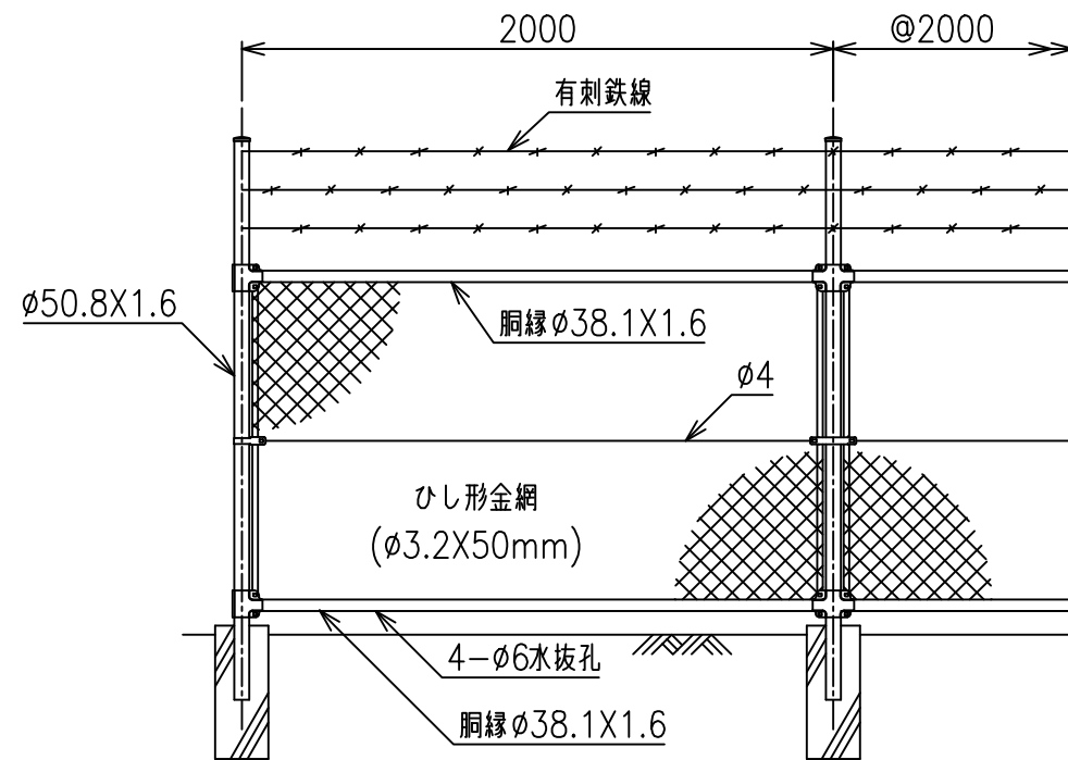
正面図 S=1/25
