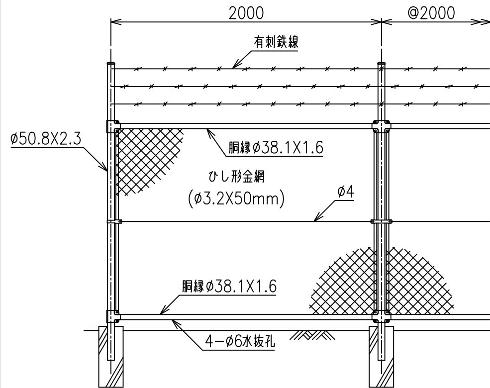
正面図 S=1/25
