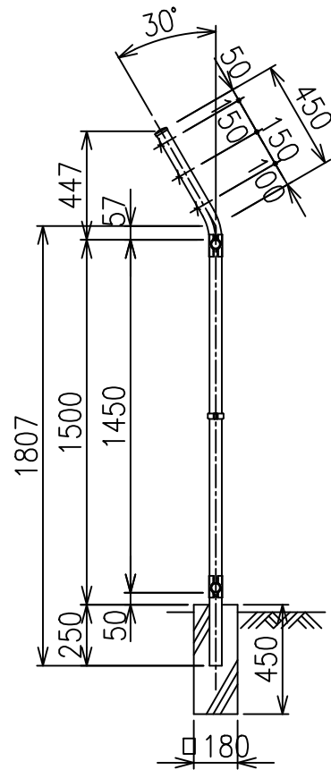
側面図 S=1/25
