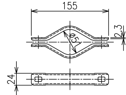
コーナー・傾斜ジョイント S=1/4
