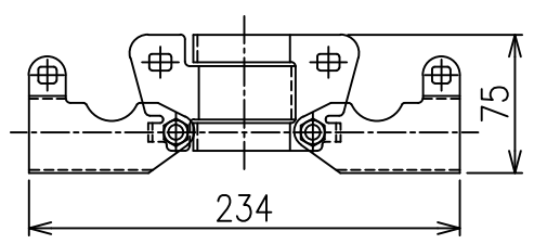
コーナー・傾斜ジョイント S=1/4
