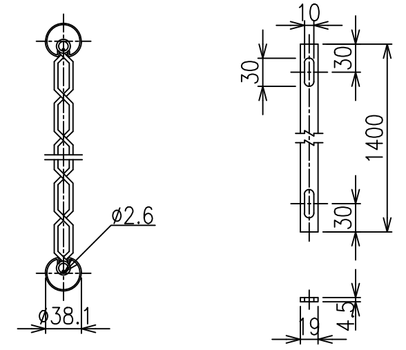
金網取付断面図 S=1/5 ストッパー S=1/5
