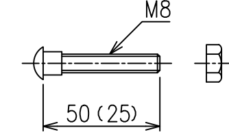
ボルトナット S=1/2 (コーナー用)
