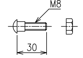
ボルトナット S=1/2
