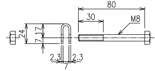
有刺鉄線取付ボルトナット S=1/2
