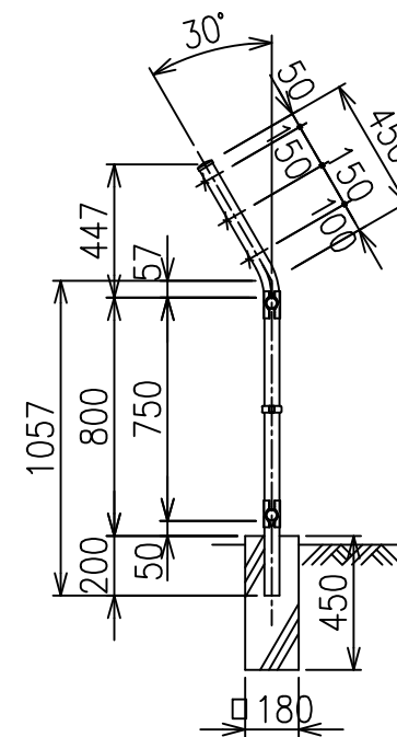
側面図 S=1/25
