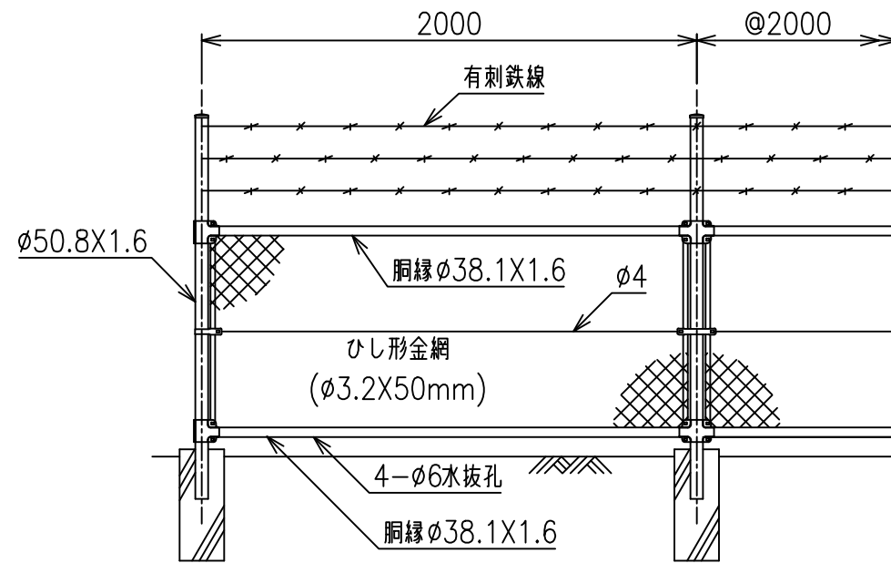
正面図 S=1/25
