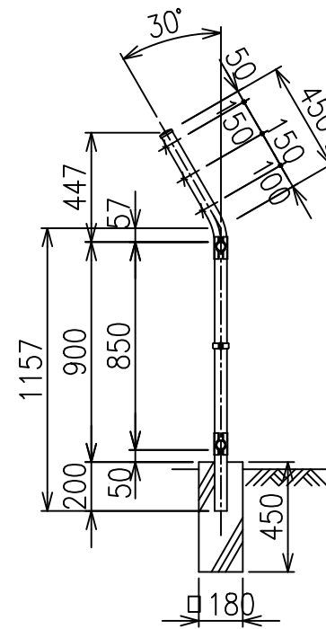
側面図 S=1/25
