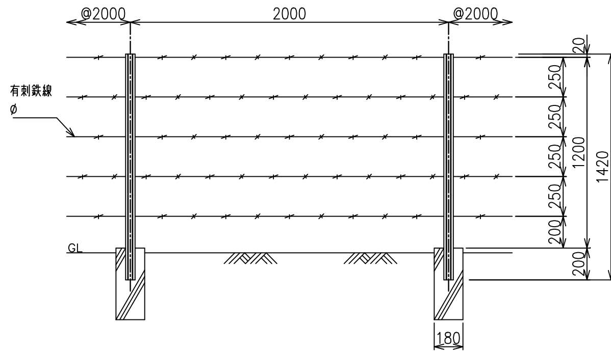
正面図 S=1/20
