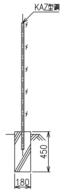
側面図 S=1/20
