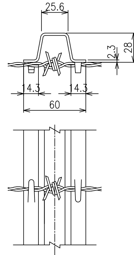
有刺鉄線取付部 S=1/2
