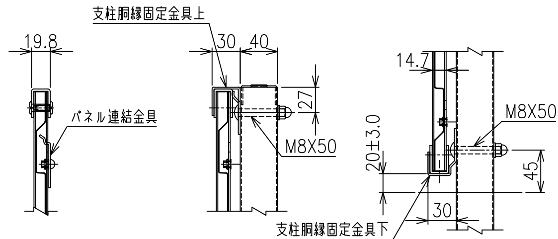
A部詳細図 S=1/4
