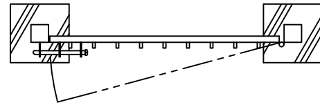
片開き門扉 S=1/20
