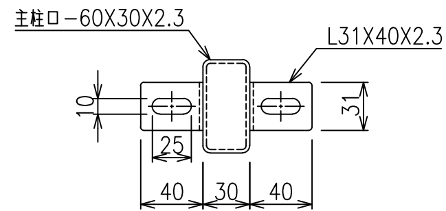
胴縁取付金具 S=1/3
