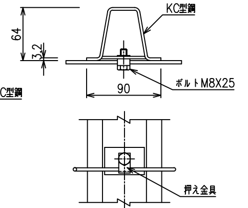
F部詳細図 S=1/3
