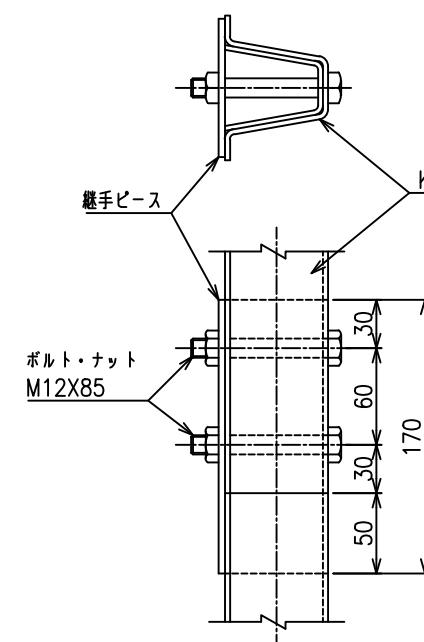
E部詳細図 S=1/3
